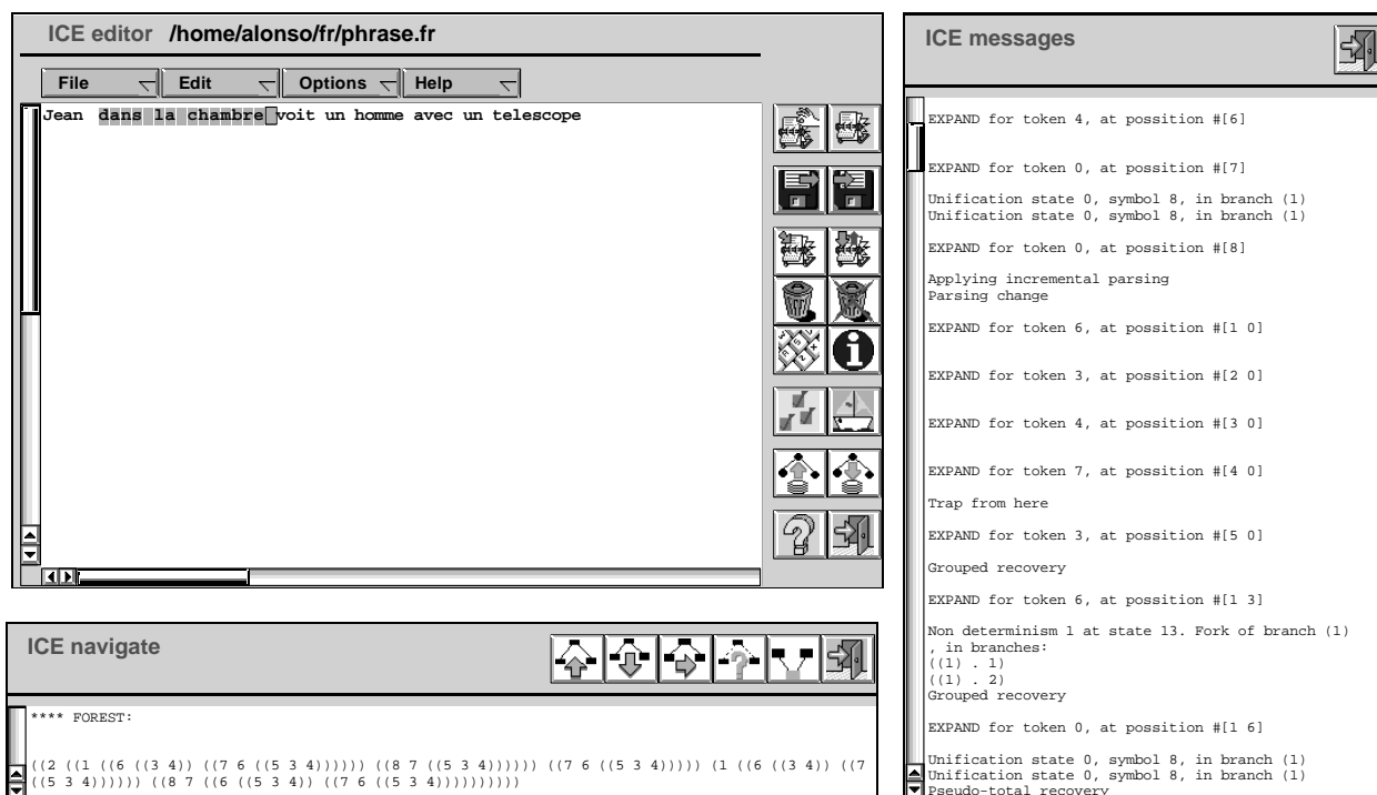
Figure 2: Environnement d'analyse de textes
