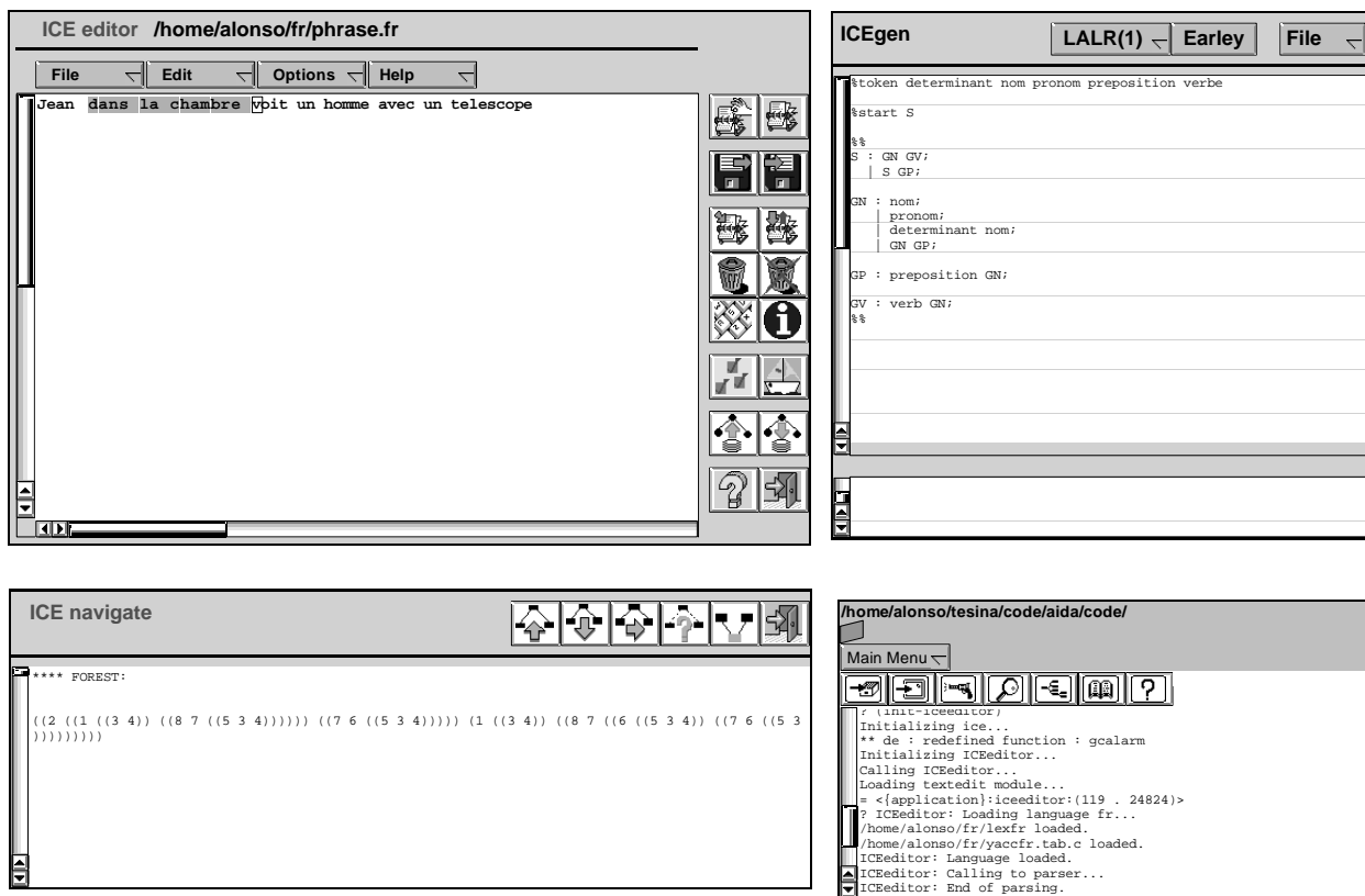
Figure 1: Environnement d'analyse de textes
