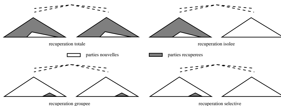
Figure 5: Types de récupération incrémentale
