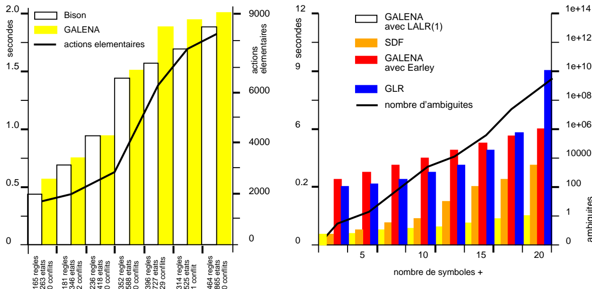
Figure 6: Temps de génération d'analyseurs et temps d'analyse
