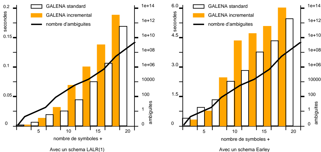
Figure 7: Résultats de l'analyse incrémentale
