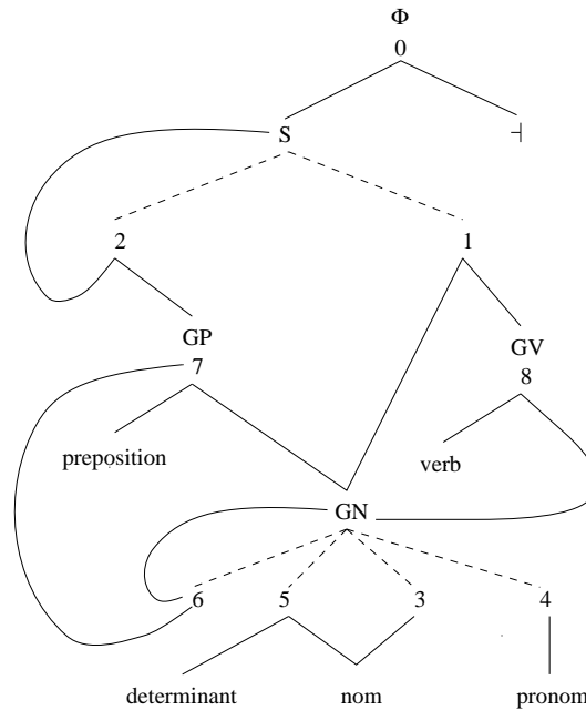
Figure 3: Graphe ET-OU de la mini-grammaire \mathcal{G}
